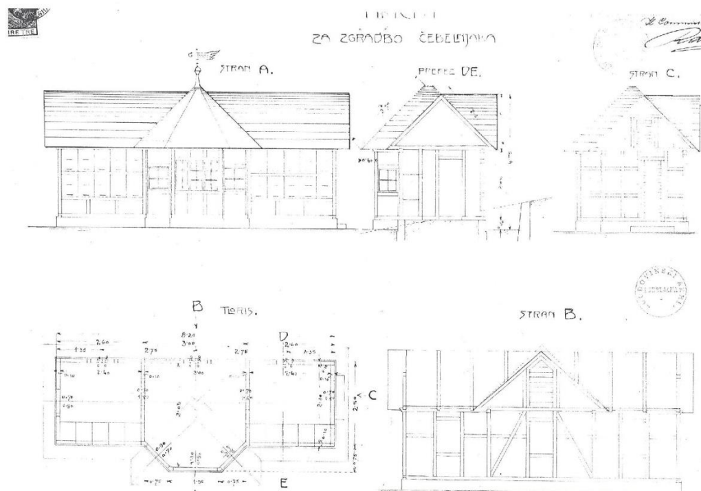
Slika 4: Načrt čebelnjaka iz leta 1925 (Zgodovinski arhiv Ljubljana, Enota v Idriji)
