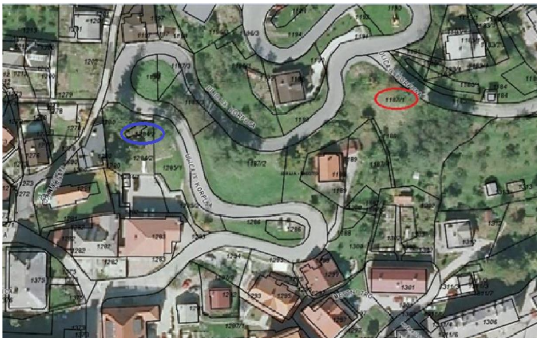
Slika 11: Načrt postavitve meščanskega čebelnjaka na nadomestno lokacijo
